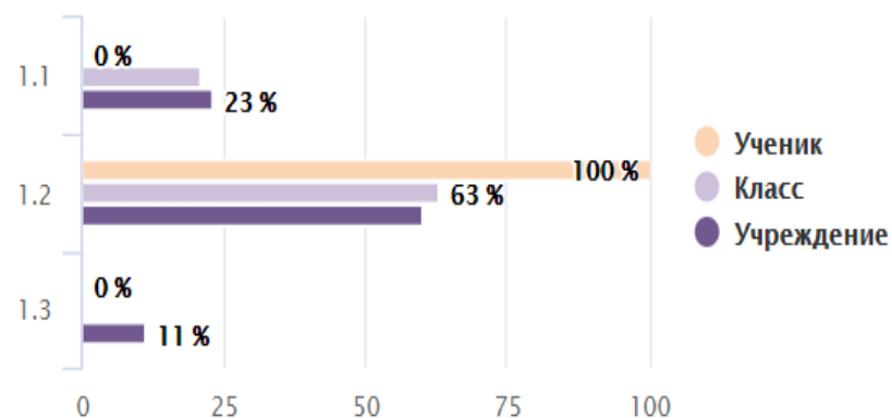
Величины и действия над ними (величинная линия)
