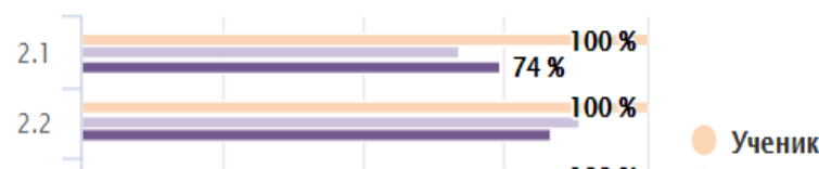
Числа и действия над ними (арифметическая линия)
